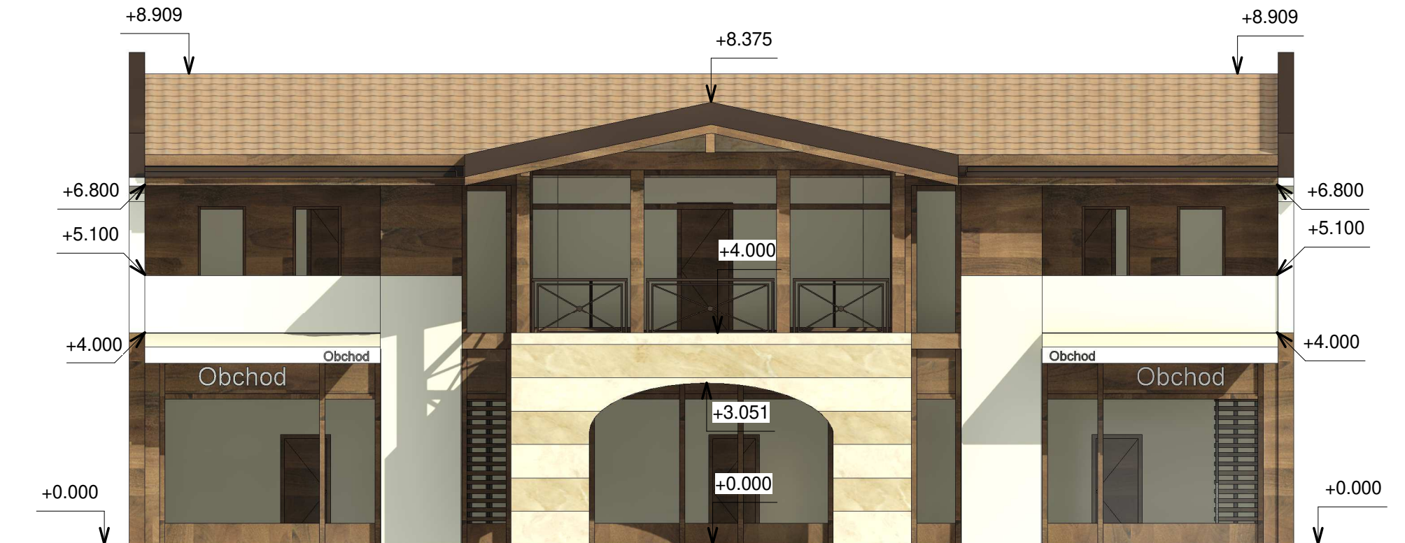
① Severovýchod 1:100
