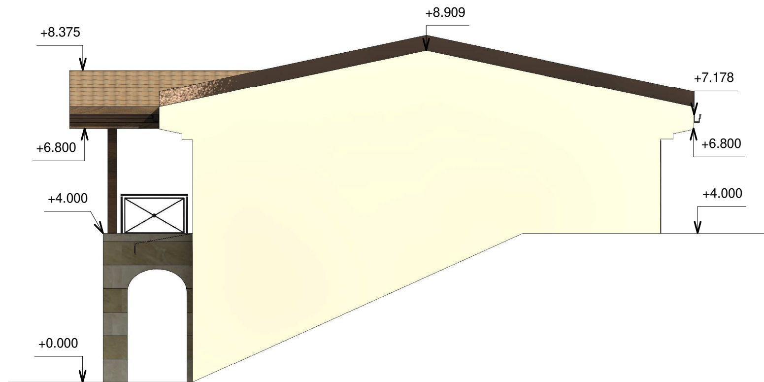
② Severozápad 1 : 100
