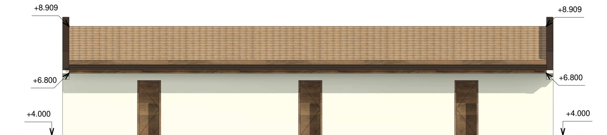
② Juhozápad 1:100
