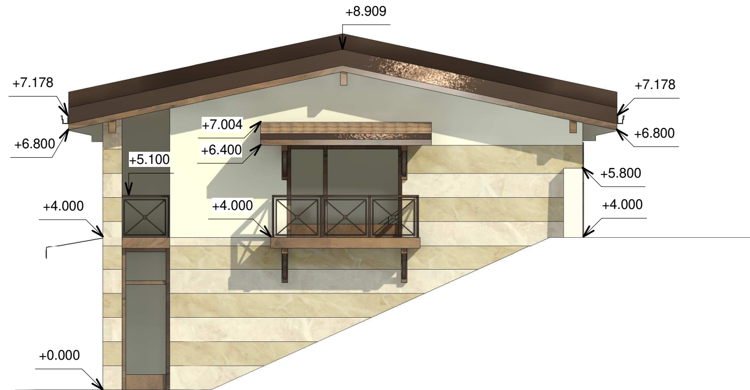
① Severozápad 1 : 100
