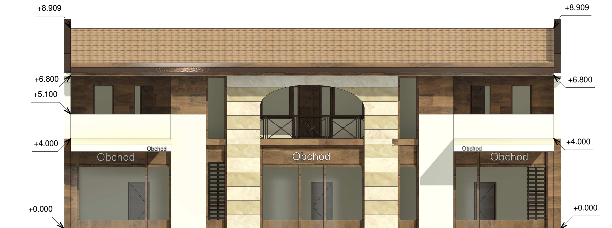
① Severovýchod 1 : 100
