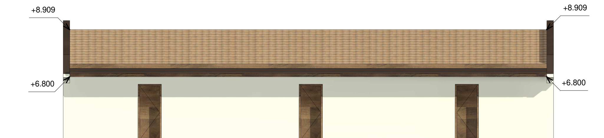
② Juhozápad 1 : 100
