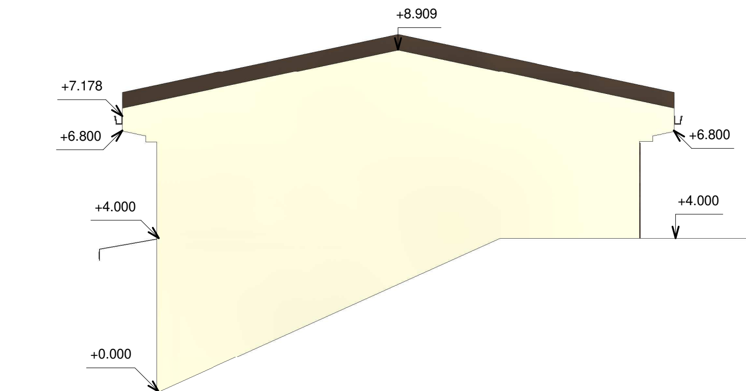
② Severozápad 1 : 100
