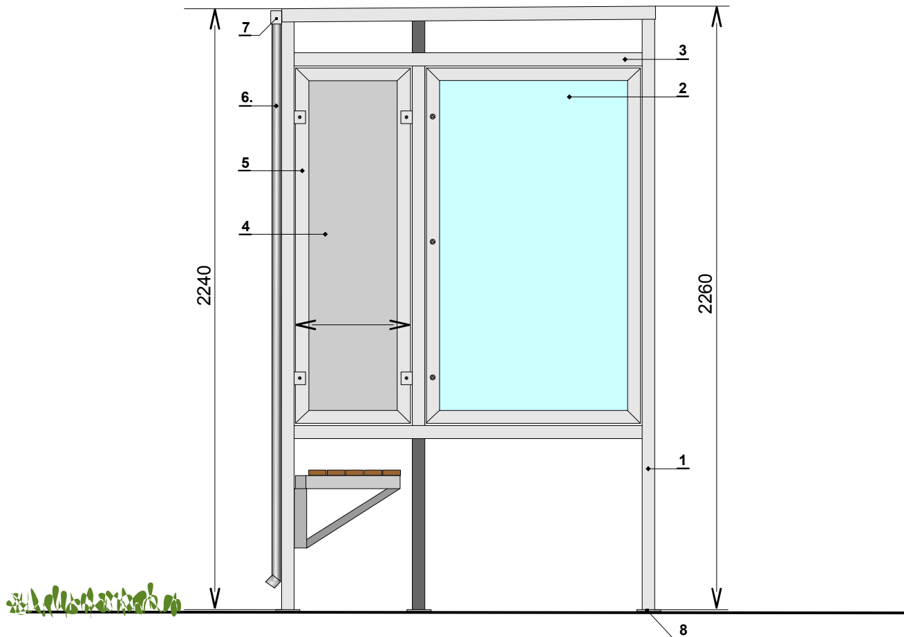
Informačný kiosk s prístreškom a lavičkou : pohľad z boku
