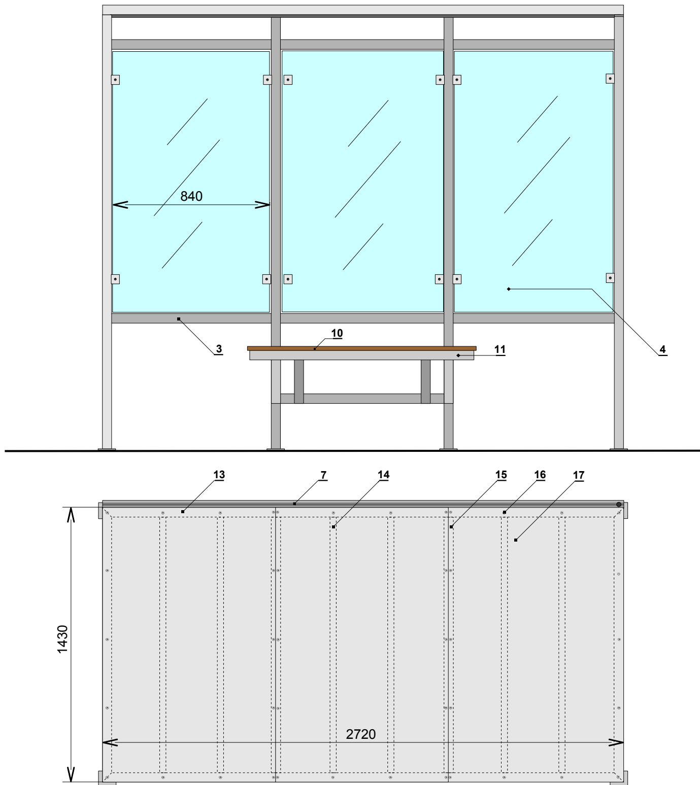
Informačný kiosk s prístreškom a lavičkou : pohľad zpredu a zhora
